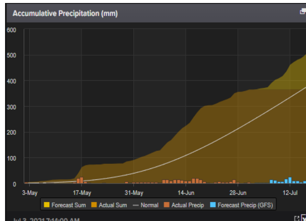
图表 12：印度马邦累计降水 GFS 模型 (mm)
