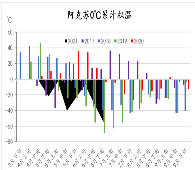
图表 1: 南疆阿克苏累计积温据平 (°C)
