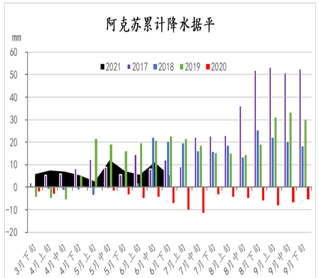
图表 2: 南疆阿克苏累计降水据平 (mm)
