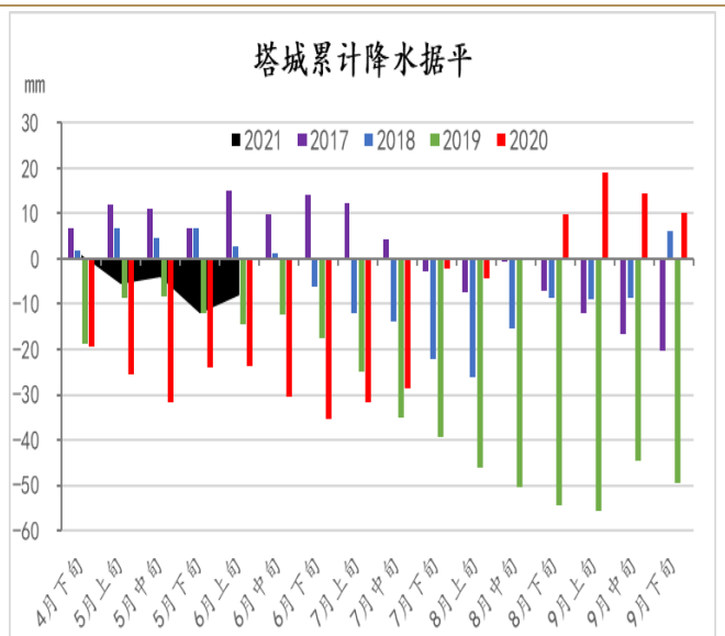
图表 4: 北疆塔城累计降水据平 (mm)
