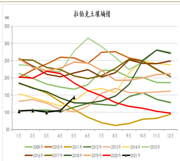
图表 5：得州拉伯克 1.6m 土壤含水率
