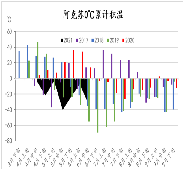
图表 1: 南疆阿克苏累计积温据平 (°C)
