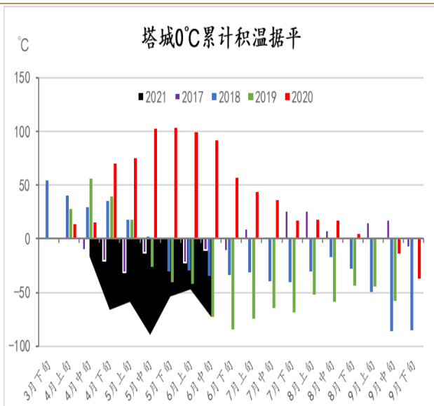
图表 3: 北疆塔城累计积温据平 (°C)
