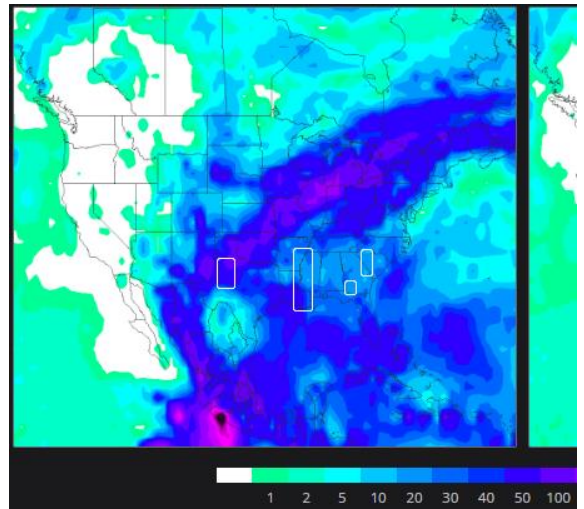
图表 8: 美国 6 月 25-7 月 2 日日降水累计量 (mm)
