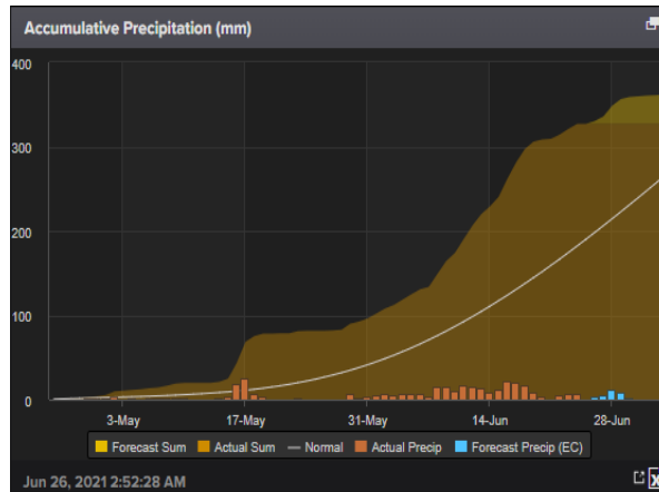
图表 12: 印度马邦累计降水 (mm)
