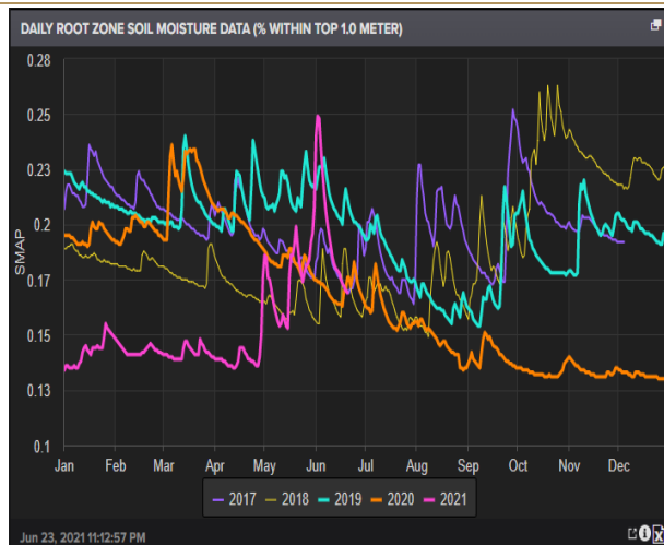
图表 3：得州拉伯克 1m 土壤含水率
