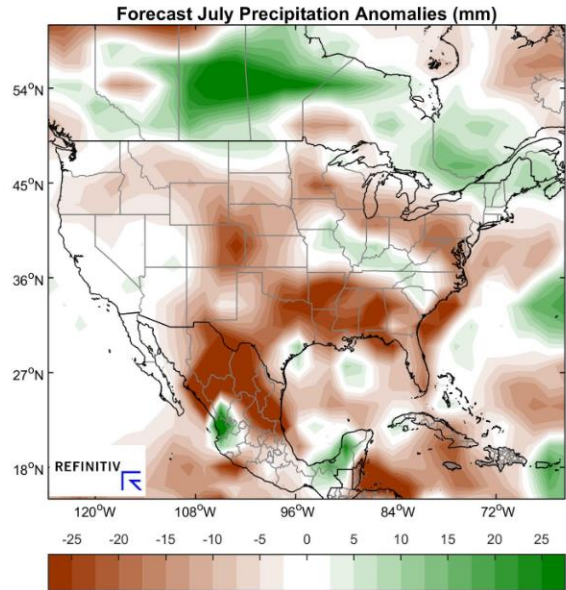
图表 10: 2021 年 7 月降水距平 (mm)
