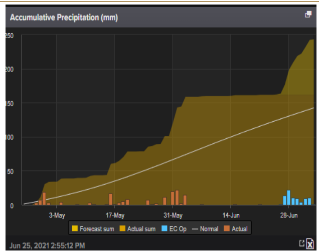
图表 4：得州拉伯克 EC 预测降水量 (mm)
