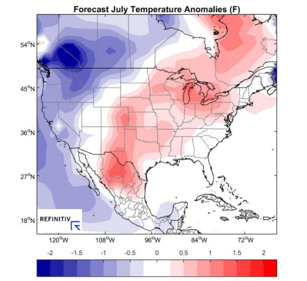
图表 9: 2021 年 7 月美国气温距平 (°F)
