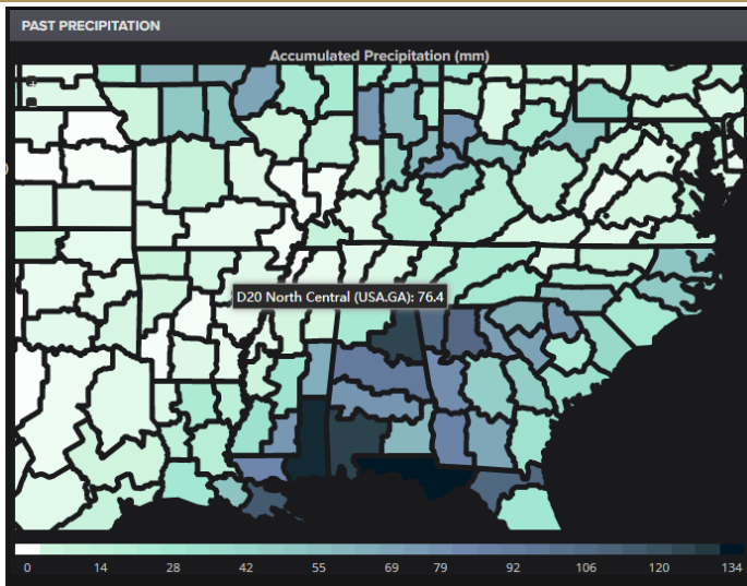
图表 7: 5月美国中南、东南棉区墒情据平
