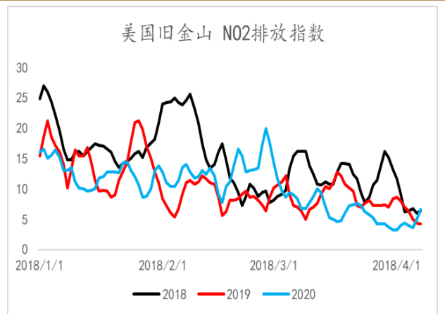
图表 32: 旧金山 N02 排放指数
