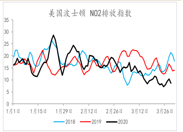
图表 30: 波士顿 N02 排放指数
