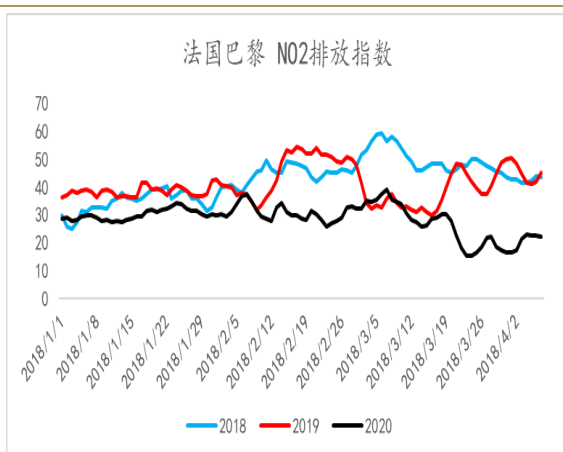
图表 9: 巴黎 NO2 排放指数
