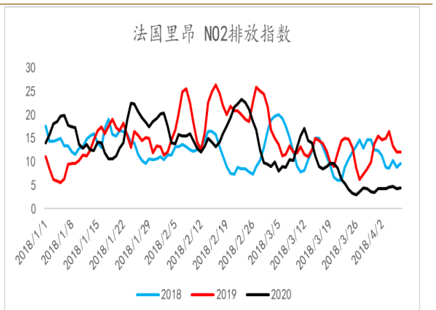
图表 10: 里昂 NO2 排放指数
