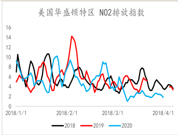
图表 29: 华盛顿 N02 排放指数
