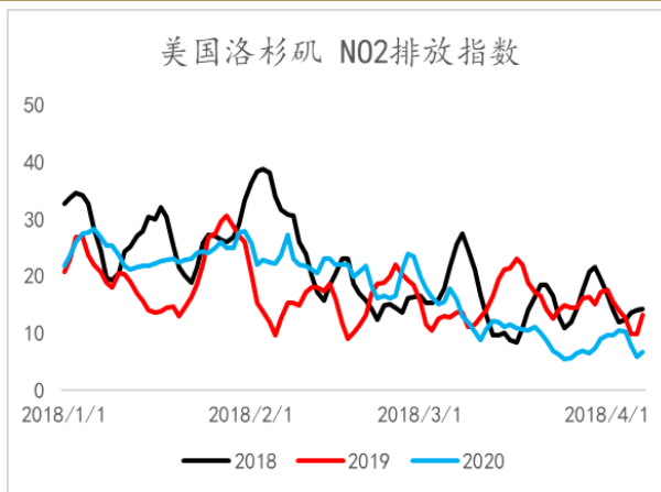
图表 31: 洛杉矶 N02 排放指数
