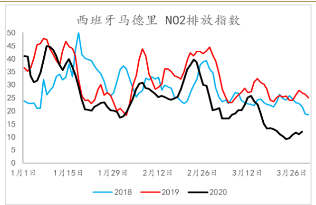
图表 6: 马德里 NO2 排放指数
