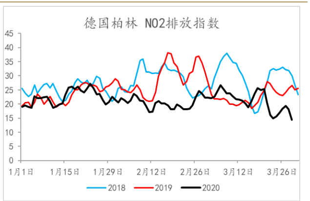
图表 8: 柏林 NO2 排放指数
